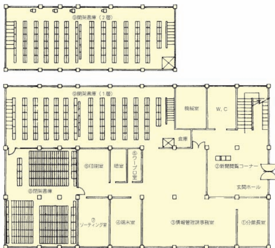
1 階平面図
