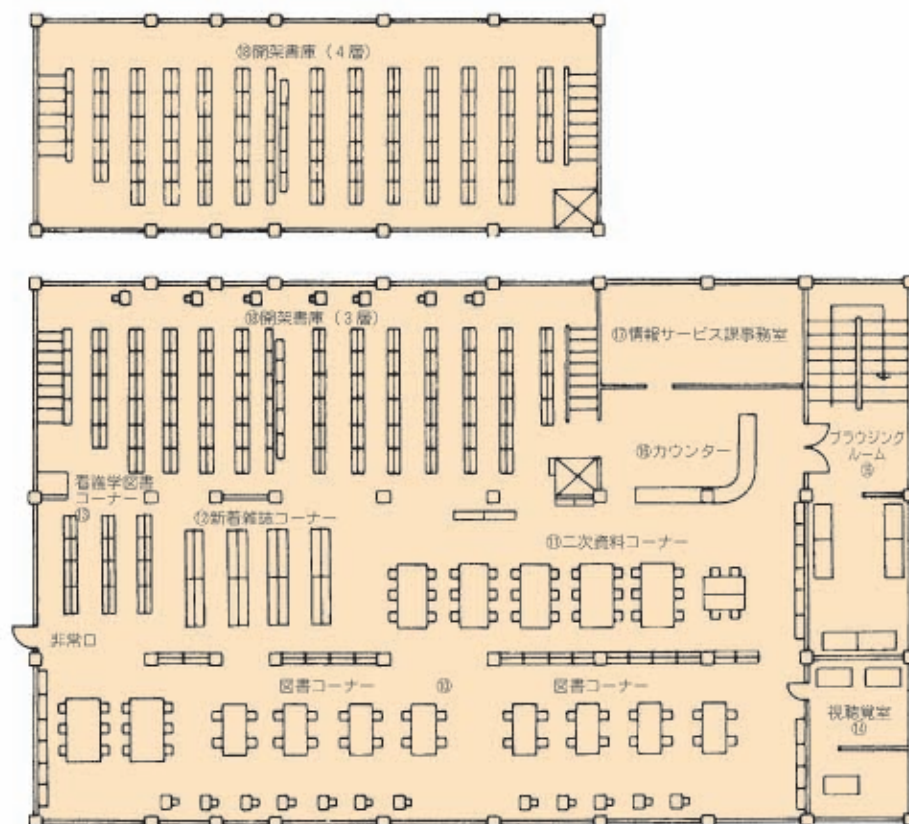
2 階平面図
