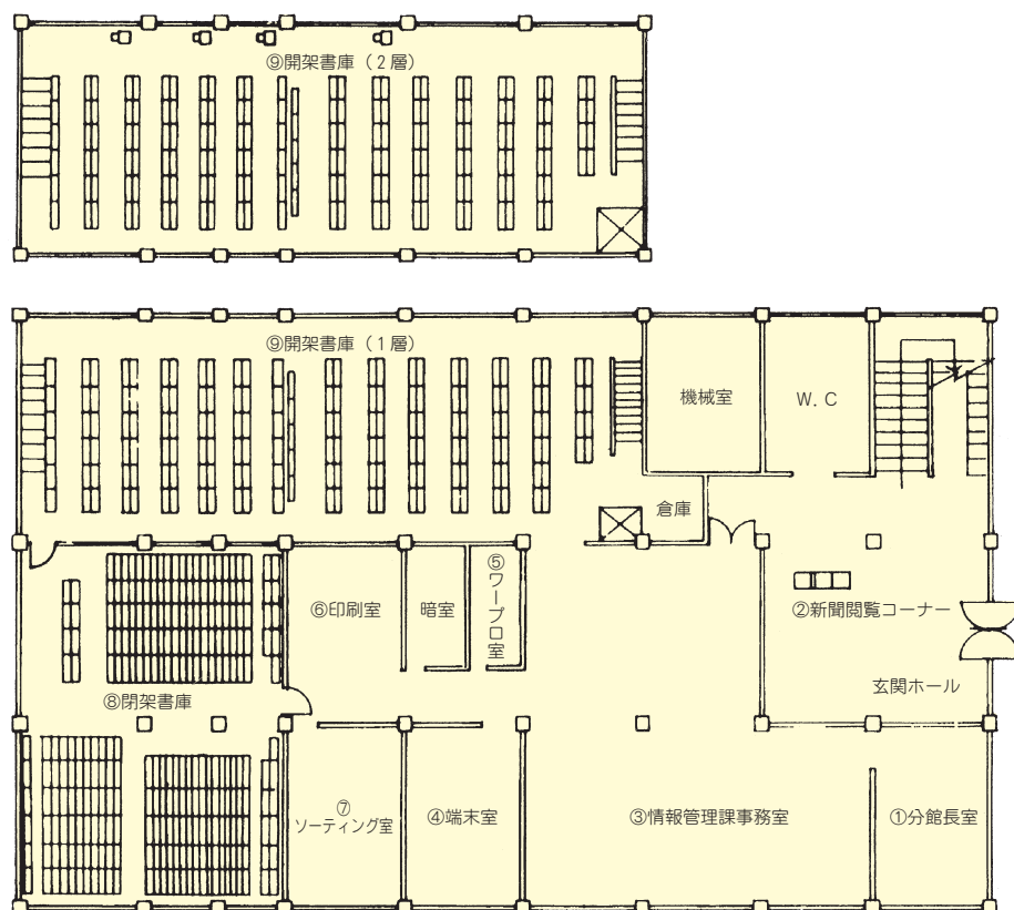
1 階 平面図
